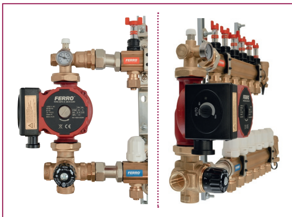
GM keverőegység felszerelése excenterrel
